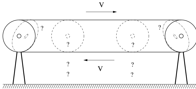
Рис. 1.20: Иллюзии ременной передачи.
