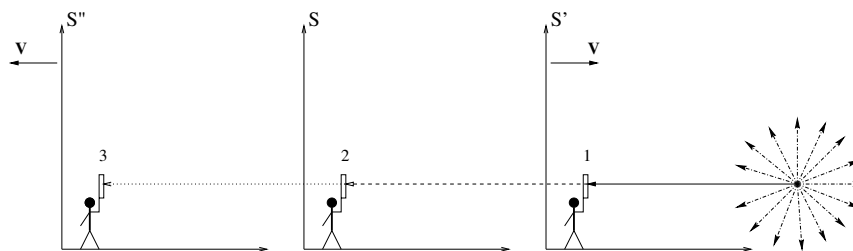
Рис. 1.16: Противоречия относительности одновременности.
