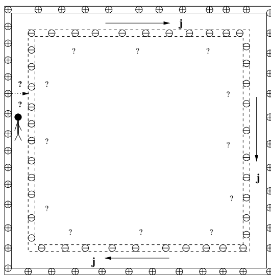
Рис. 1.32: Парадокс рамки с током.
