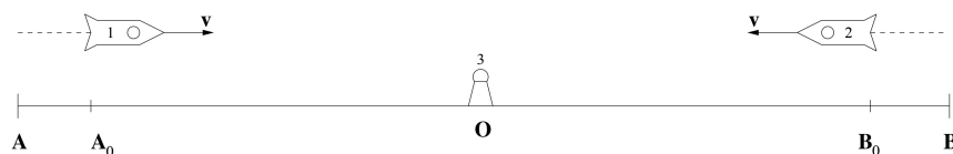
Рис. 1.2: Модифицированный парадокс близнецов.
