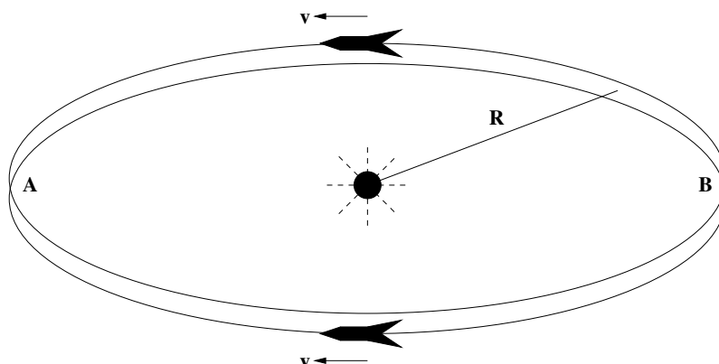
Рис. 1.10: Движения по круговым орбитам.
