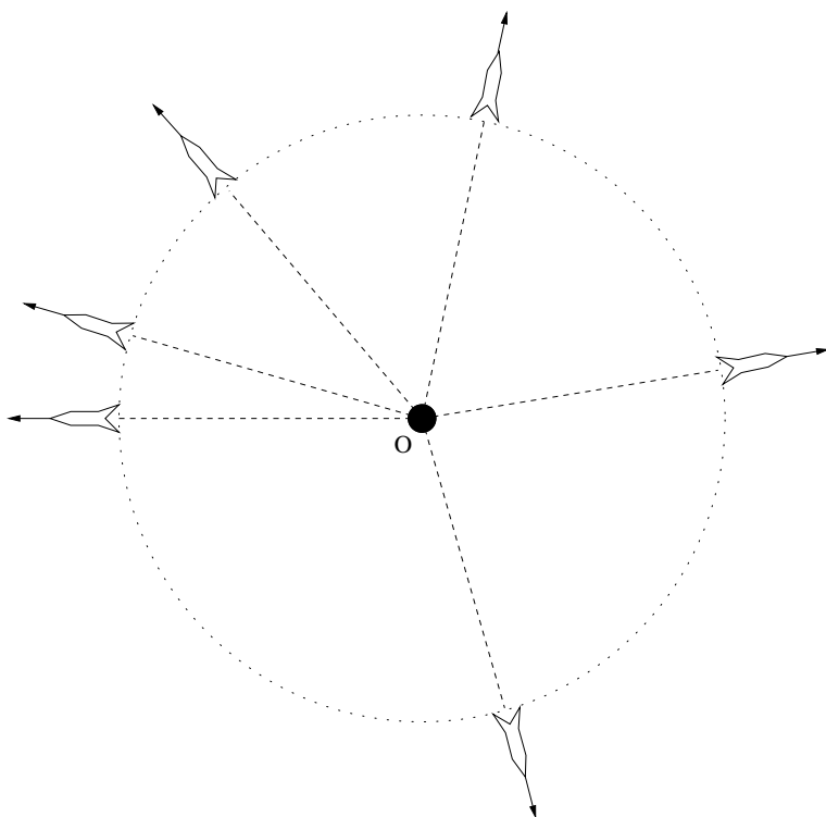
Рис. 1.3: Парадокс п близнецов.
