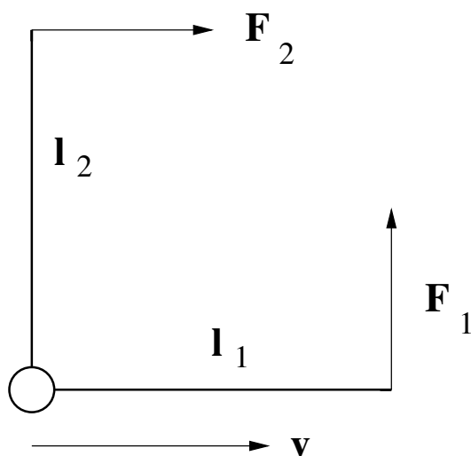
Рис. 4.10: Парадокс рычага.
