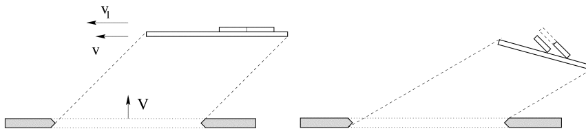
Рис. 1.24: Парадокс скользящих стержней.
