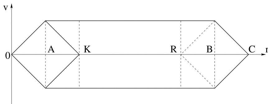
Рис. 1.1: Роль ускорений в парадоксе близнецов.
