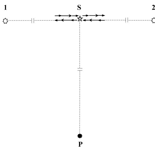
Рис. 1.31: Релятивистские фантазии про аберрацию.
