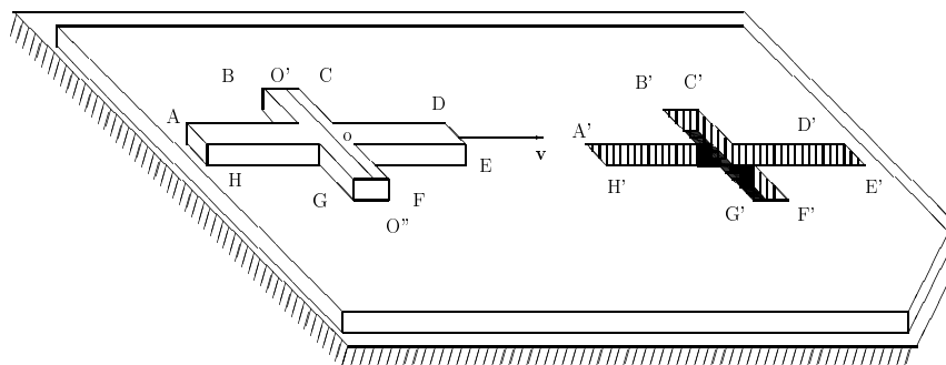
Рис. 1.19: Парадокс креста.
