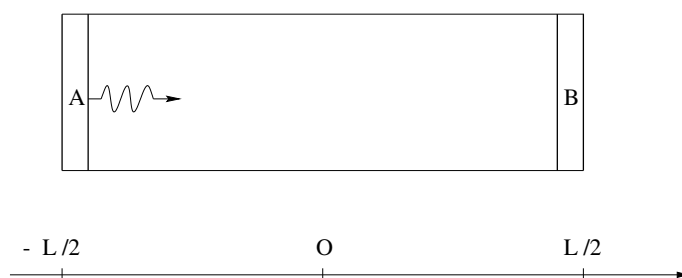
Рис. 4.11: Связь массы излучения с её энергией.
