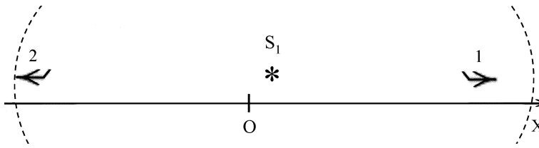
Рис. 1.28: Обмен сигналом.
