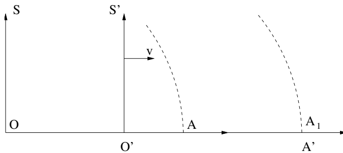
Рис. 1.29: Парадокс нелокальности.
