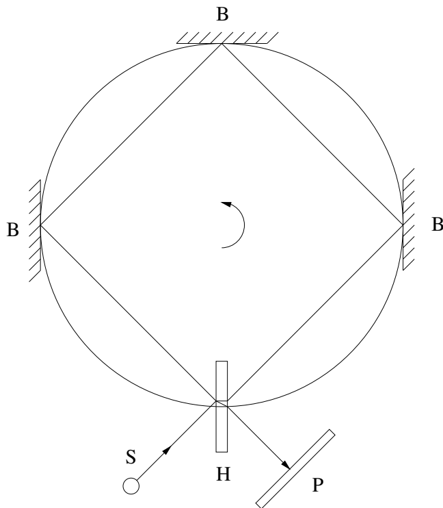
Рис. 3.4: Опыт Саньяка.
